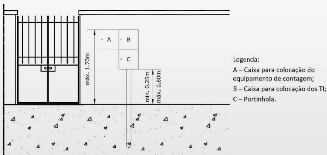
Figura 5.13 – Ligação em Baixa Tensão Especial (BTE)
