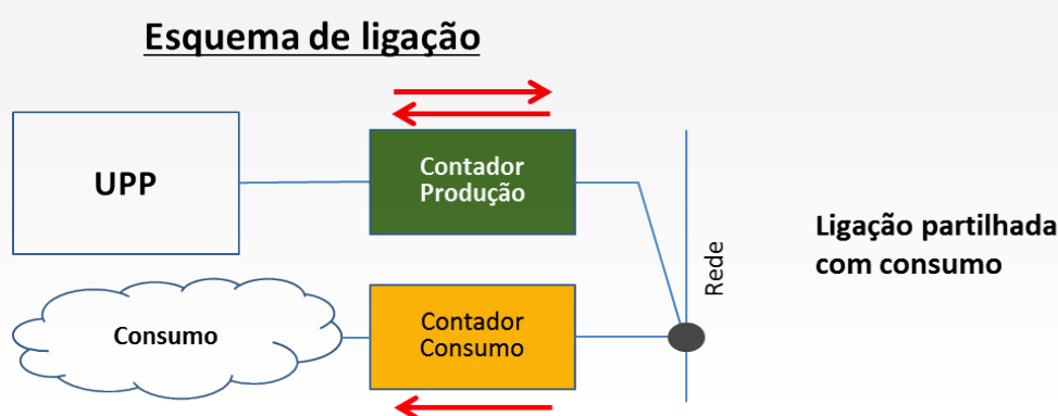
Figura 9.3 – Esquema tipo de ligação à rede de uma Unidade de Pequena Produção
