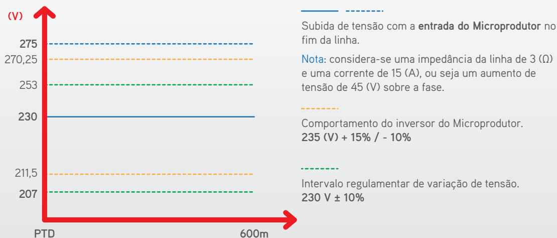
Figura 0.1 – Diagramas do perfil da tensão numa rede de distribuição BT 600 m
