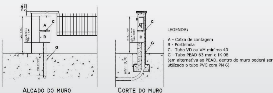
Figura 5.8 – Ligação a partir de rede subterrânea de uma instalação dotada de muro com altura suficiente [DIT-C14-100]
