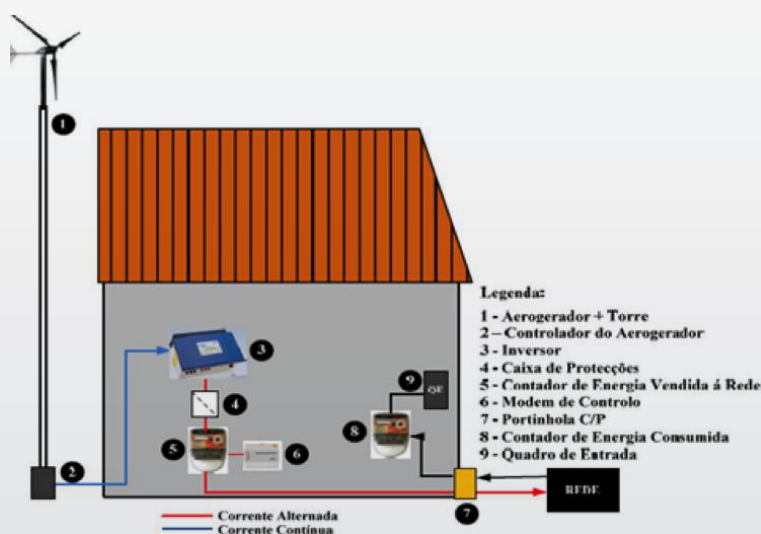
Figura 9.6 – Esquema simplificado de um sistema de Microprodução eólico ligado à rede de distribuição
