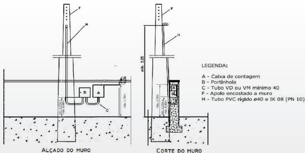
Figura 5.6 – Ligação a partir de rede aérea de uma instalação unifamiliar dotada de muro sem pilar
