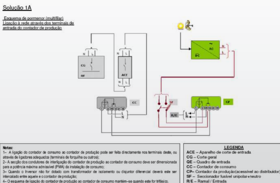
Fig 6 – Cliente BT com Miniprodução / UPP em BT (solução 1A)
