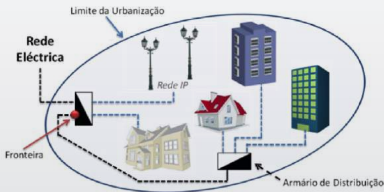
Figura 8.4 – Ligação à Rede Eléctrica de uma Urbanização, através de linha subterrânea
