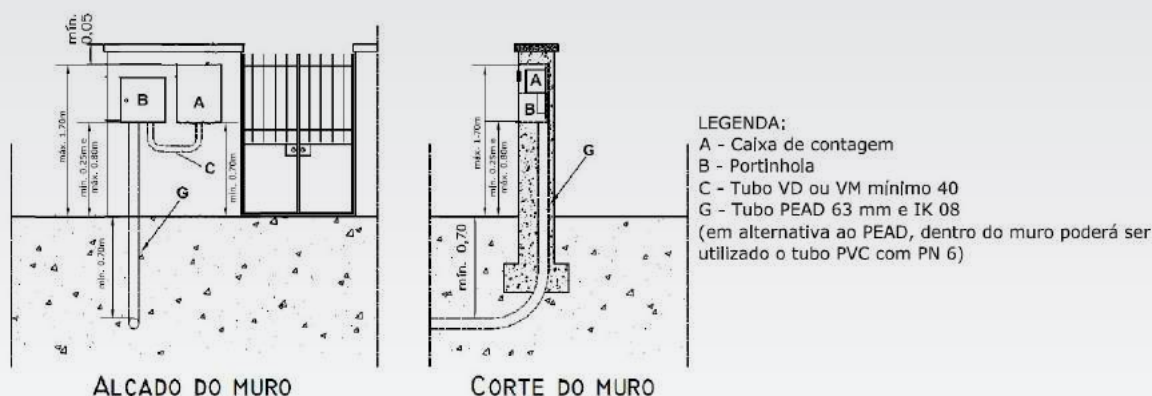
Figura 5.9 – Ligações a partir de rede subterrânea de uma instalação dotada de muro sem altura suficiente [DITC14-100]
