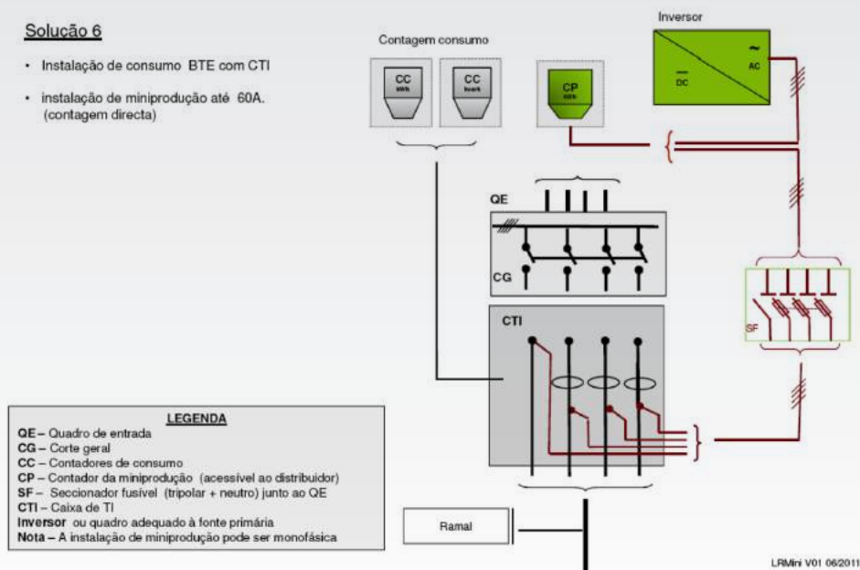
Fig 11 - Cliente BTE com Miniprodução / UPP em BT \leq 41,4 kVA (solução 6)
