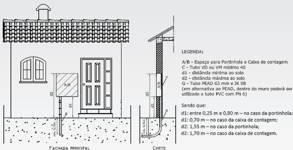
Figura 5.11 – Ligação a partir de rede subterrânea de uma instalação sem muro [DIT-C14-100]
