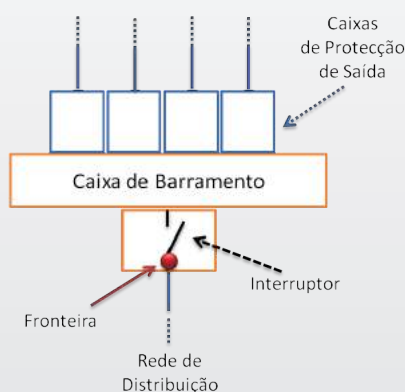
Figura 5.3 - Ponto de fronteira entre a Rede Pública e a Instalação Coletiva (sem Portinhola > 400 A)
