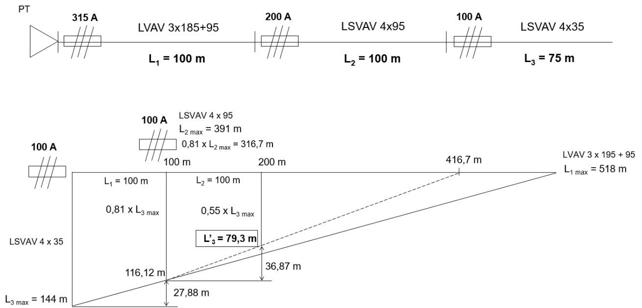
Figura C4 – Exemplo de aplicação da metodologia de cálculo geométrico, i.e., Regra do Triângulo.
