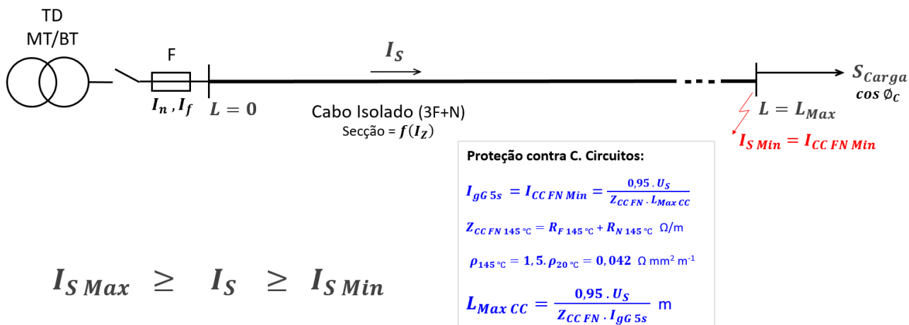
Figura C2 – Dimensionamento da proteção fusível na condição de corrente de defeito fase-neutro mínima (ICC FN Min) de atuação da proteção.
