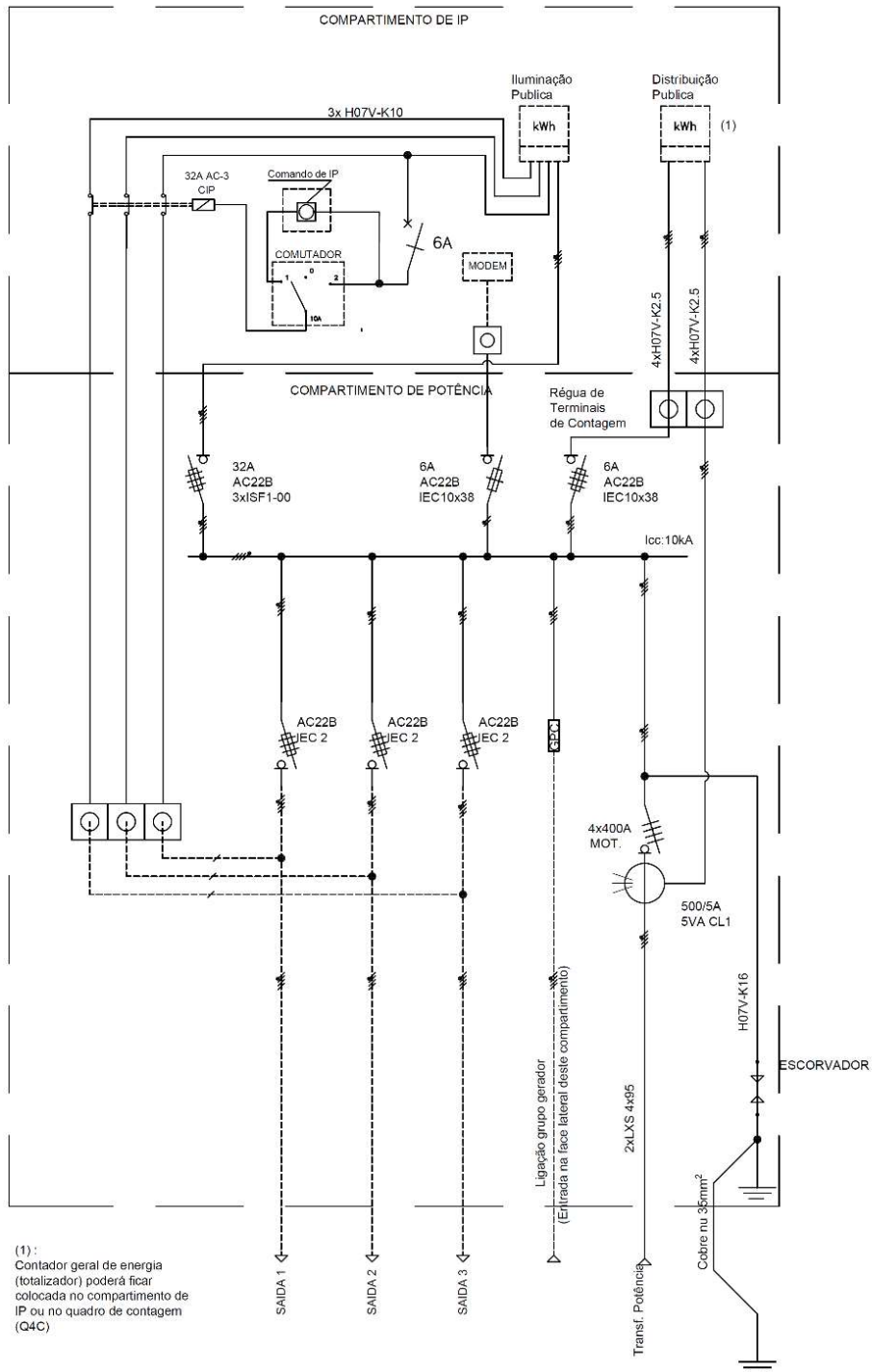
Figura 2 – Esquema elétrico unifilar do quadro (QGBT de uso exclusivo pelo ORD)
