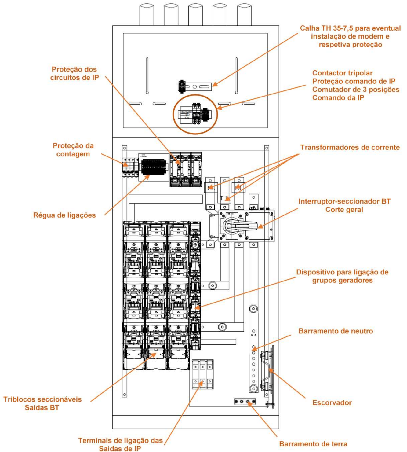
Figura 3 – Disposição exemplificativa dos equipamentos no quadro
