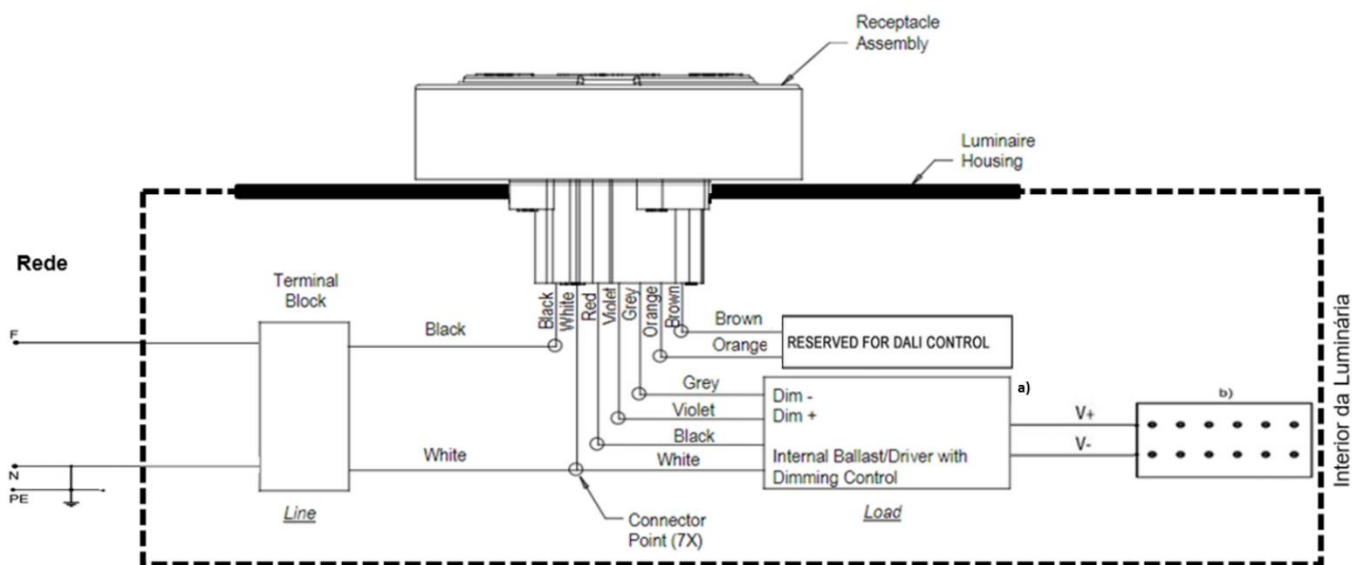
Figura A.3 - Luminária com tecnologia LED e regulação de fluxo através de comando por tensão contínua 0-10 Vdc - aplicação na rede subterrânea
