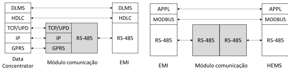
Figura 2 – Pilhas protocolares da comunicação DTC–EMI (à esquerda) e HEMS–EMI (à direita, opcional)
