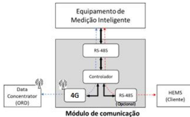
Figura 1 - Arquitetura do módulo de comunicação
