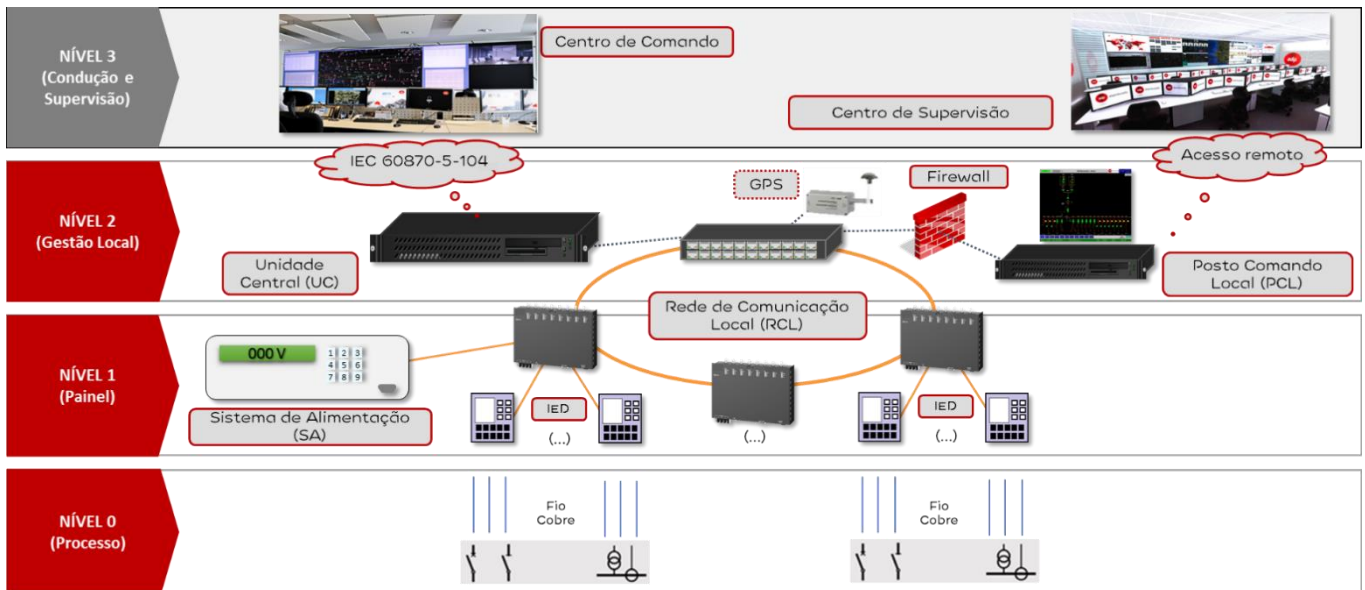
Figura 1 – Arquitetura do SPCC de uma subestação AT/MT.
